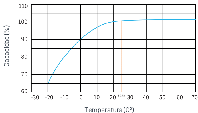
Efectos de la temperatura sobre la capacidad a 0,5 °C
