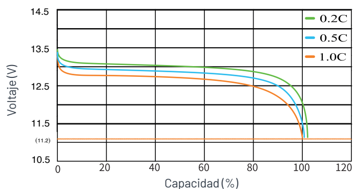
Rendimiento de descarga a 25°C
